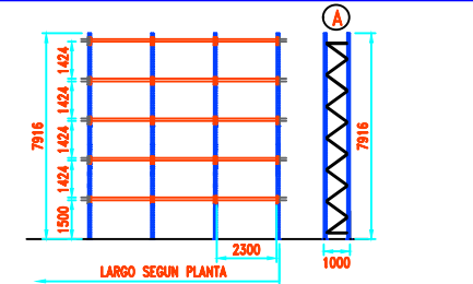
ELEVACION DE RACKS SELECTIVOS A
