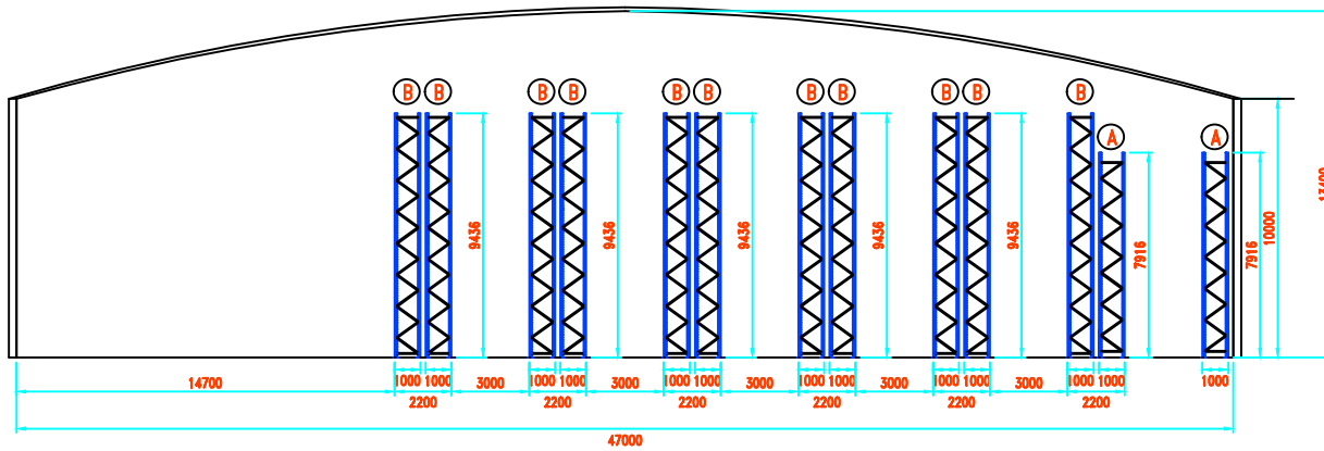
ELEVACION DE RACKS SELECTIVOS A
