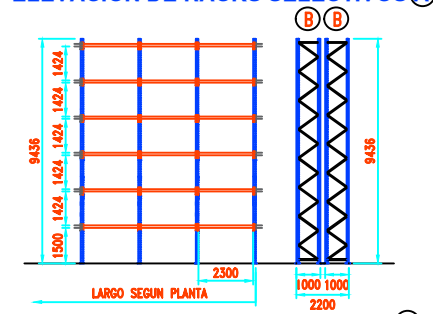
ELEVACION DE RACKS SELECTIVOS B
